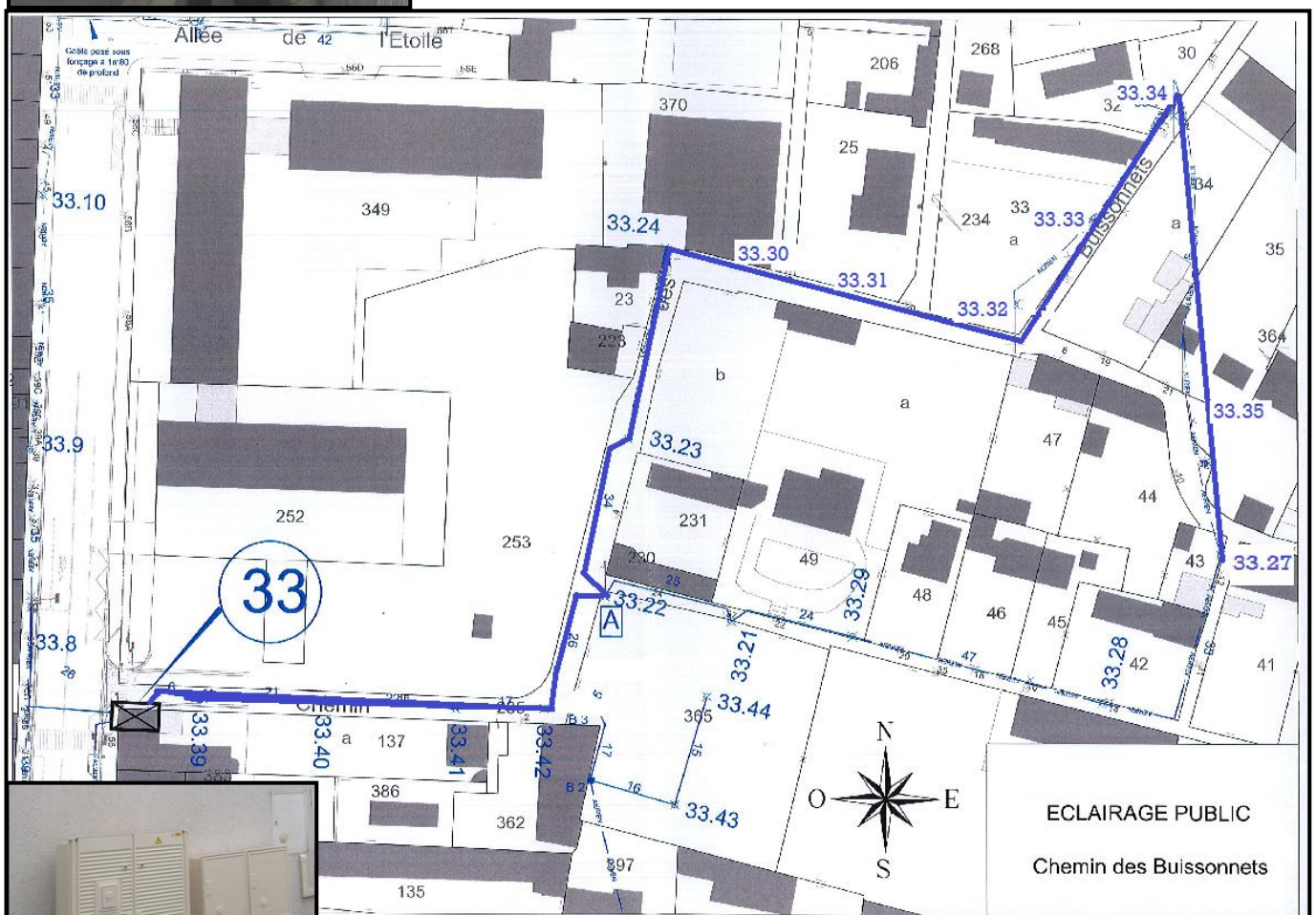
Plan du projet éclairage
