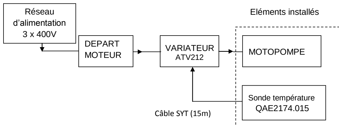
Schéma de principe du groupe motopompe de recyclage
