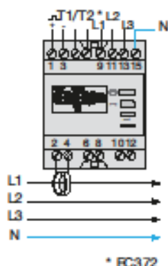
Comptage en réseau triphasé équilibré
