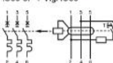
iC60 3P + Vigi iC60
