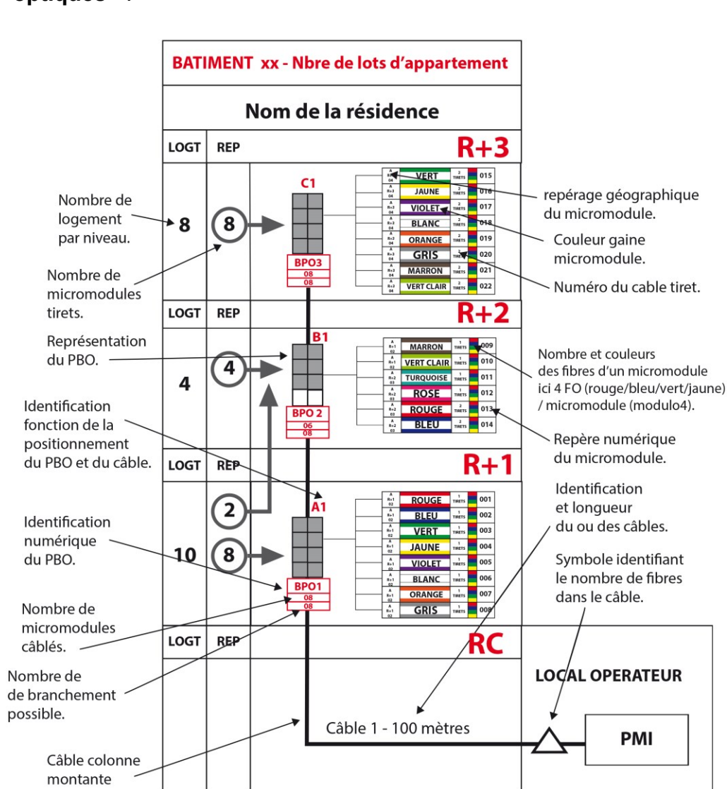
Code couleur et rang des fibres optiques (exemple d'un câble micromodule 48 FO modulo 4)
